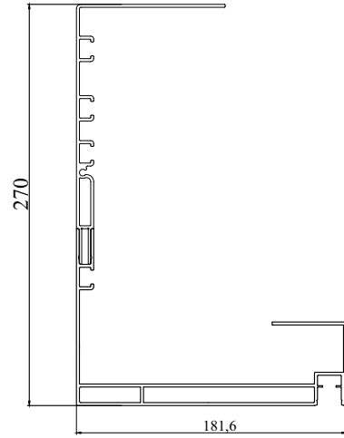
GRONDA
