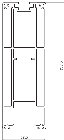
GUIDA
