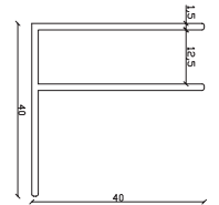
BACCHETTA TETTUCCIO
