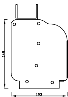
FLANGIA CASSONETTO
