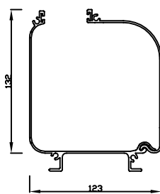
CASSONETTO
